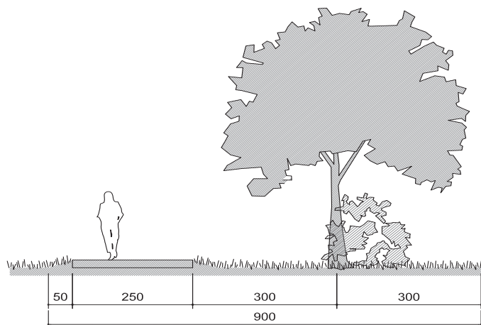
PERCORSO CON FILARE ARBOREO (acquisizione aree = 9,00m)
