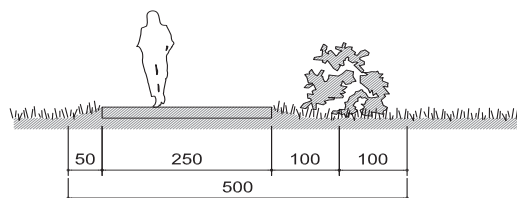
PERCORSO CON SIEPE (acquisizione aree = 5,00m)
