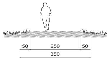
PERCORSO SEMPLICE (acquisizione aree = 3,50m)
